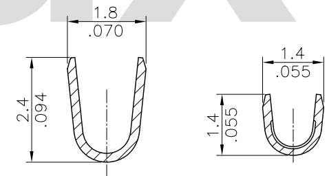
A-A SEC.
